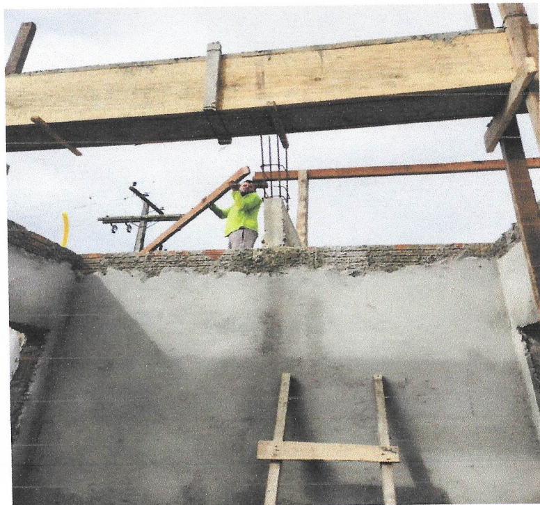
Foto 37- EXECUÇÃO DO TELHADO
