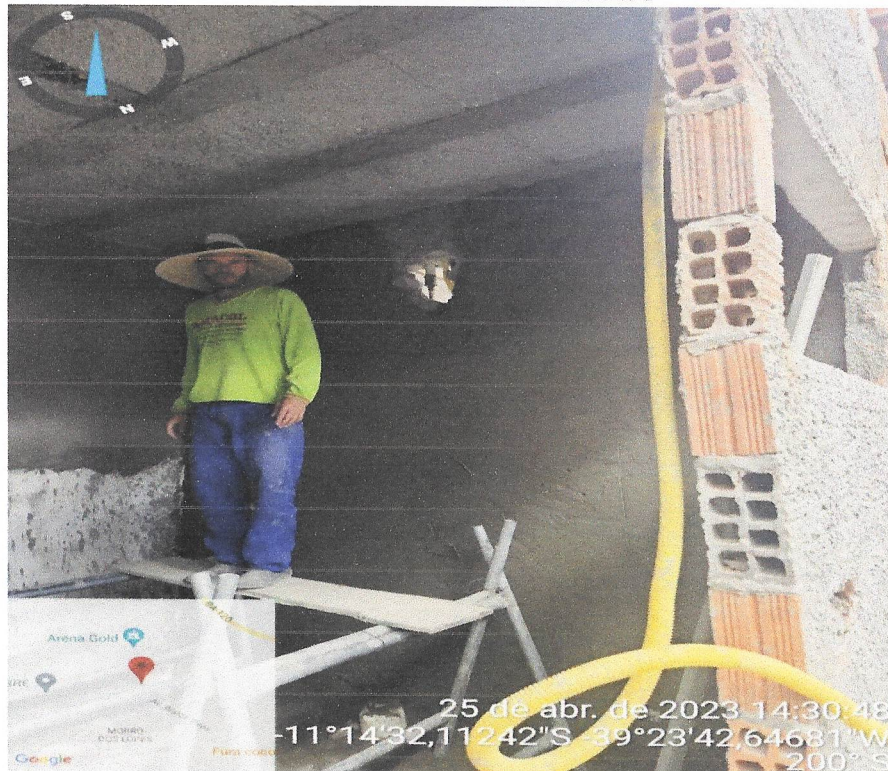
Foto 14- REBOCO DA ALVENARIA.
