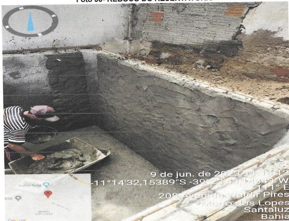
Foto 30- REBOCO DO RESERVATÓRIO
