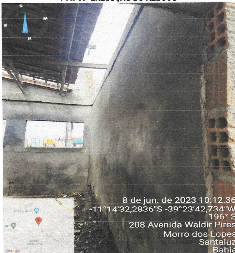
Foto 36- EXECUÇÃO DO REBOCO
